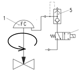
Bild 4 - Wirkbild bei Ausführung mit Magnetventil – die Sicherheitsstellung ist – Ventil zu – Die Feder hält die Armatur geschlossen
