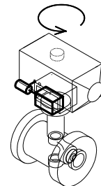
Bild 5 - Wirkbild bei Ausführung mit Magnetventil und Schnellentlüftung – die Sicherheitsstellung ist – Ventil zu – Die Feder hält die Armatur geschlossen
