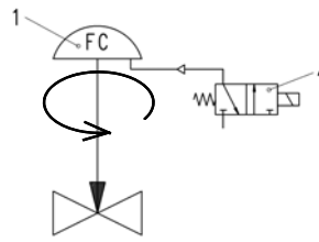
Bild 4 - Wirkbild bei Ausführung mit Magnetventil – die Sicherheitsstellung ist – Ventil zu – Die Feder hält die Armatur geschlossen
