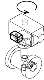
Bild 4 - Wirkbild bei Ausführung mit Magnetventil – die Sicherheitsstellung ist – Ventil zu – Die Feder hält die Armatur geschlossen
