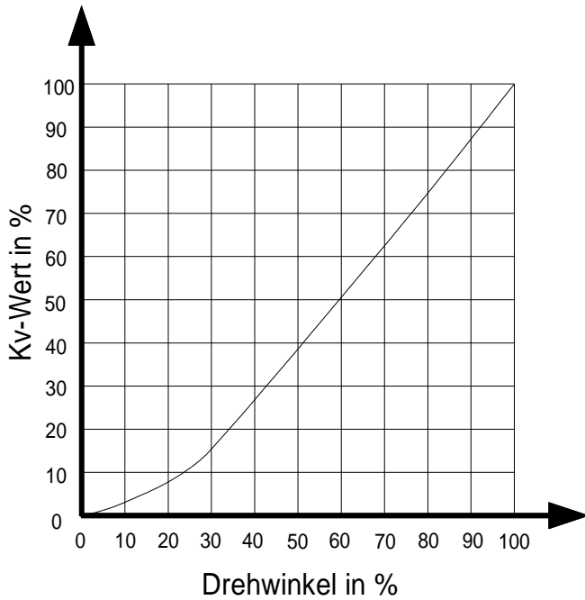
Bild 8 Natürliche Kennlinie
