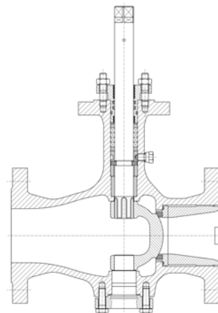
Bild 7 weich dichtend, Anströmung von hinten – Medium schließt
