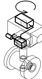
Bild 6 - Wirkbild bei Ausführung mit Magnetventil, Schnellentlüftung und Stellungsregler – die Sicherheitsstellung ist – Ventil zu – Die Feder hält die Armatur geschlossen
